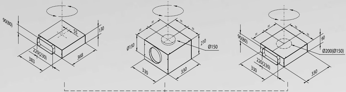
KIT MOTORE E1300
